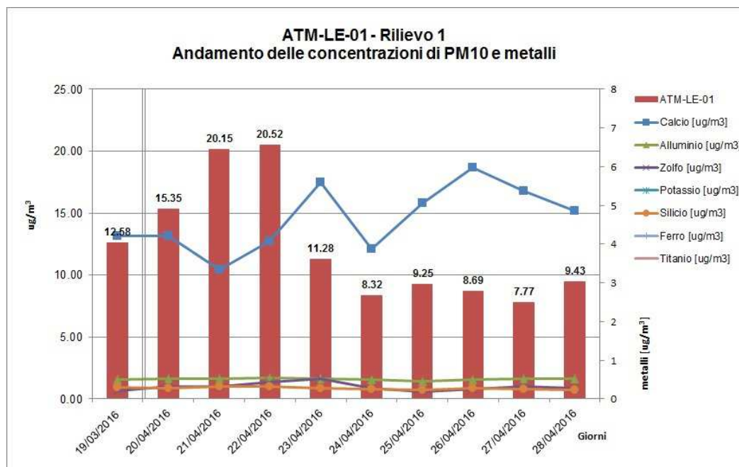
Fig. 2.2/B – Andamento delle concentrazioni di PM10 e di metalli terrigeni rilevate presso la postazione ATM-LE-01 dal 19/03/2016 al 28/04/2016 (si considerano solo gli effettivi giorni di campionamento)
