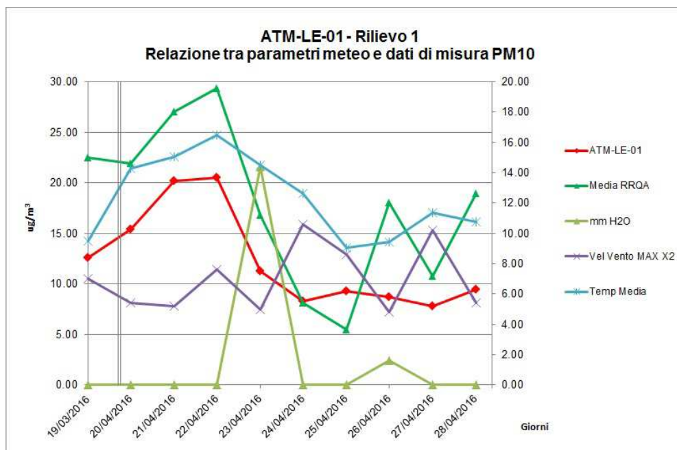
Fig. 2.2/F – Andamento delle concentrazioni di PM10 e dei parametri meteo presso la postazione ATM-LE-01 e presso le centraline ARPA dal 19/03/2016 al 28/04/2016 (si considerano solo gli effettivi giorni di campionamento)
