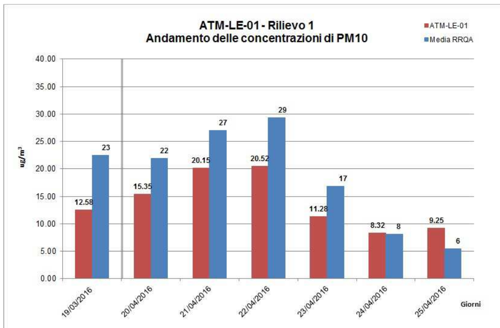
Fig. 2.2/E – Andamento delle concentrazioni di PM10 presso la postazione ATM-LE-01 e presso le centraline ARPA dal 19/03/2016 al 28/04/2016 (si considerano solo gli effettivi giorni di campionamento)
