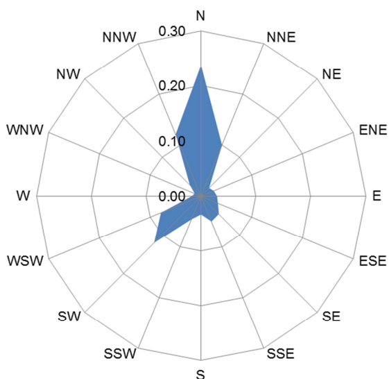
Fig. 2.1/G – Andamento della rosa dei venti, costruita sulla base dei dati rilevati presso la stazione di monitoraggio ATM-LE-01 (periodo 19/03/16 – 28/04/16, si considerano solo gli effettivi giorni di campionamento)
