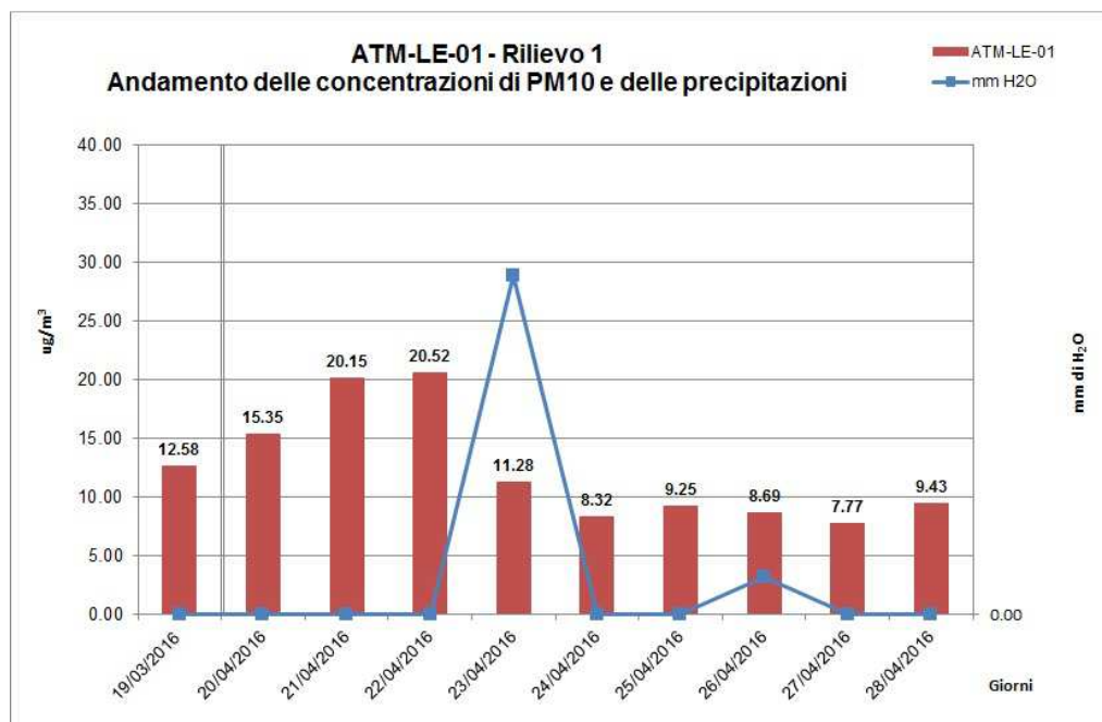
Fig. 2.2/A – Andamento delle concentrazioni di PM10 e delle precipitazioni rilevate presso la postazione ATM-LE-01 dal 19/03/2016 al 28/04/2016 (si considerano solo gli effettivi giorni di campionamento)
